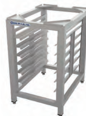
SHEC-611 830 × 705 × 520 mm Capacidad / Capacity / Capacité / Kapazität 6 × GN 1/1 – 6 × 600 × 400
